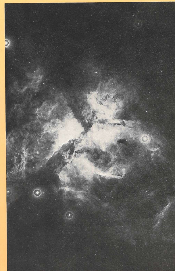
The Eta Carina Nebula. (Cerro Tololo photo)
